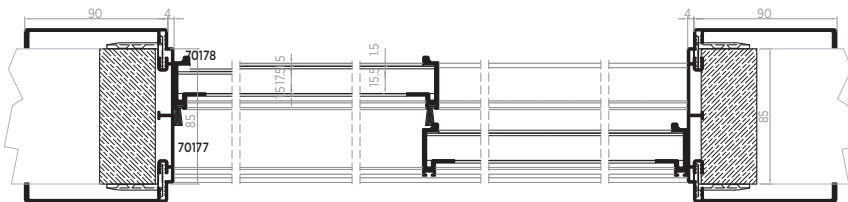
SECCIÓN LONGITUDINAL PANEL JAPONÉS JAPANESE PANEL LONGITUDINAL SECTION
