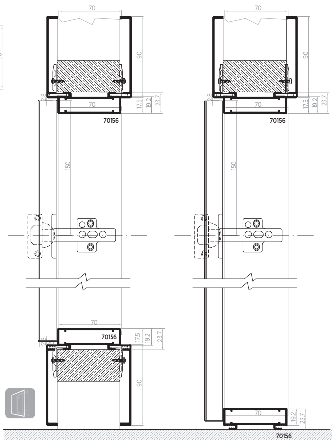
SECCIÓN TRANSVERSAL CON TAPAJUNTAS INFERIORES CROSS SECTION WITH BOTTOM FLASHINGS
