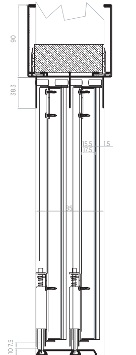
SECCIÓN TRANSVERSAL SIN TAPAJUNTAS INFERIORES CROSS SECTION WITHOUT BOTTOM FLASHINGS
