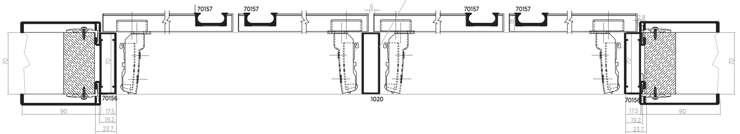
SECCIÓN LONGITUDINAL 4 HOJAS 4 SASHES LONGITUDINAL SECTION
