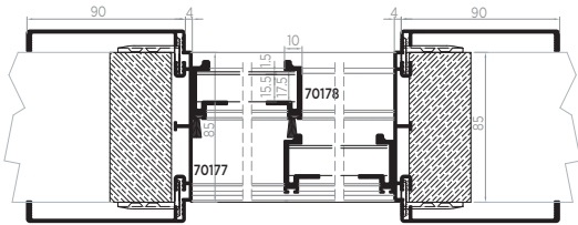
SECCIÓN LONGITUDINAL LONGITUDINAL SECTION
