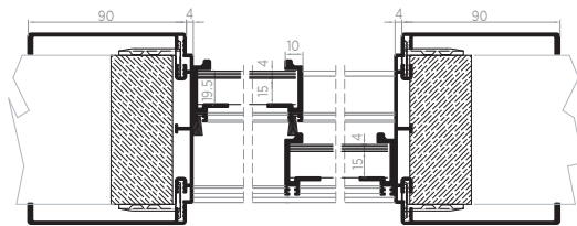
SECCIÓN LONGITUDINAL ESPEJO MIRROR LONGITUDINAL SECTION
