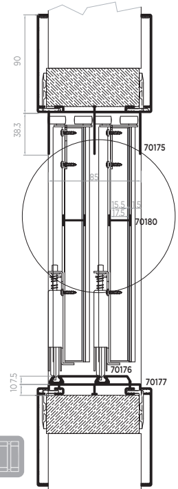
SECCIÓN TRANSVERSAL PANEL JAPONÉS JAPANESE PANEL CROSS SECTION
